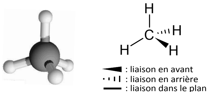
FIGURE 7 – Molécule de méthane : modélisation 3D et représentation de Cram
