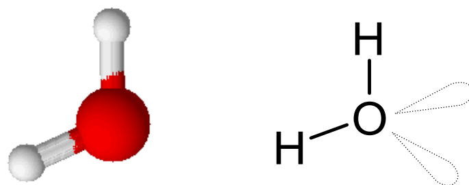
FIGURE 9 – Molécule d'eau : modélisation 3D et représentation de Cram
