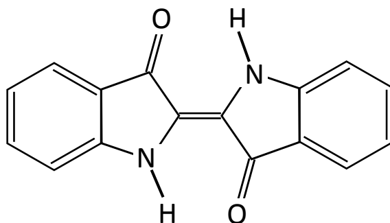
FIGURE 6 – Molécule d'indigo
