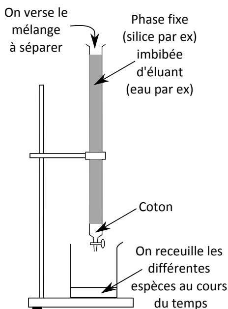
FIGURE 4 – chromatographie sur colonne
