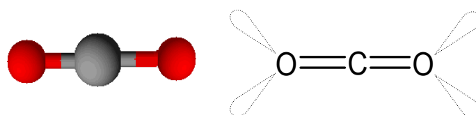
FIGURE 10 – Molécule de dioxyde de carbone : modélisation 3D et représentation de Cram
