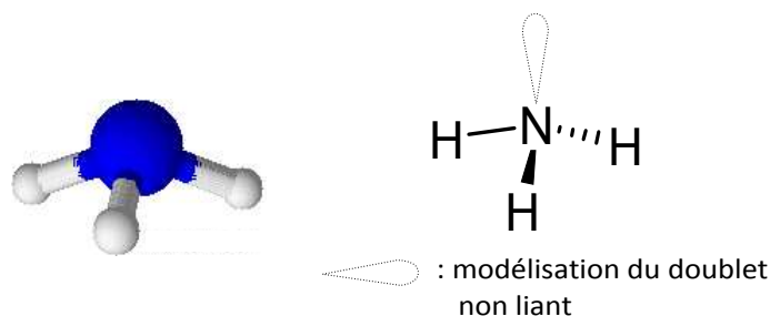
FIGURE 8 – Molécule d'ammoniac : modélisation 3D et représentation de Cram
